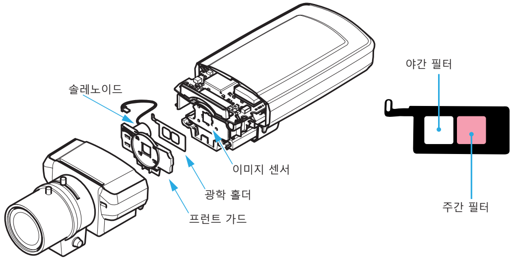
그림 3: 적외선 차단 필터와 주야간 카메라 내 위치. 주간 모드에서, 적색 필터를 사용해 적외선이 카메라 센서에 도달하지 못하게 함
