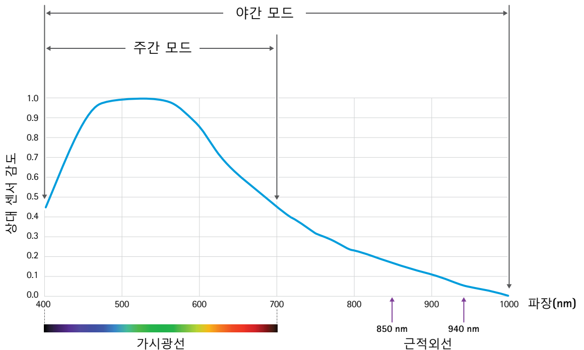
그림 2: 비주얼 카메라 센서의 상대 감광도를 보여주는 다이어그램. 주야간 카메라가 주간 모드일 때, 가시광선만 센서에 도달합니다. 야간 모드의 경우, 가시광선과 최저 적외선 범위의 적외선이 센서에 도달하고 영상 구현에 사용됩니다.
