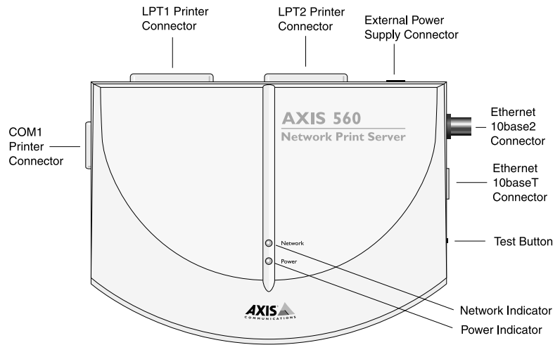
Skizze des AXIS 560
