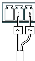
Netzeingang, 20–24 V Wechselstrom AXIS P5512: max. 23,5 VA
