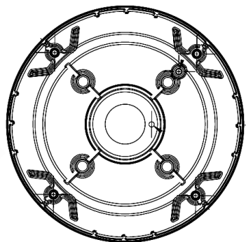
Adaptateur de suspension (Vue de dessous)
