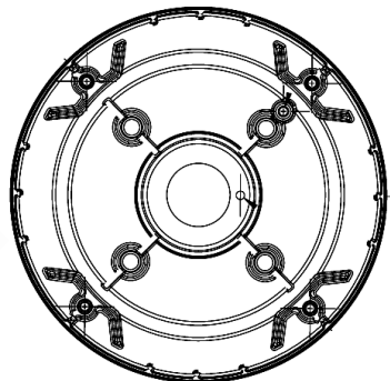
Adattatore per soffitti (vista inferiore)
