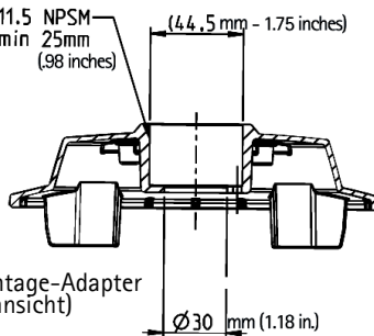
Hängemontage-Adapter (Untenansicht)
