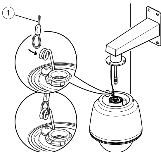
Exemple de montage (support mural vendu séparément)
