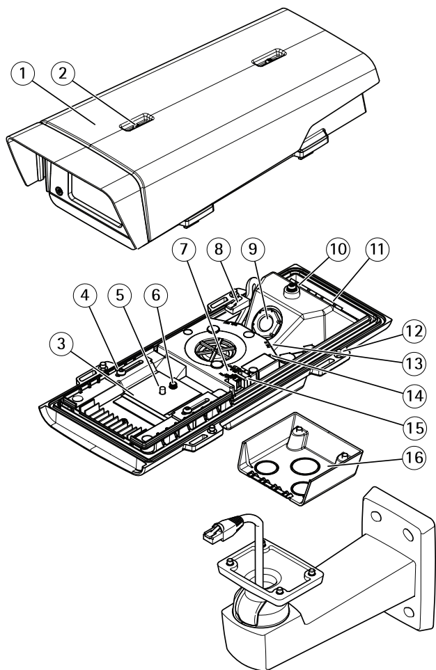
AXIS T92E20-Schutzgehäuse
