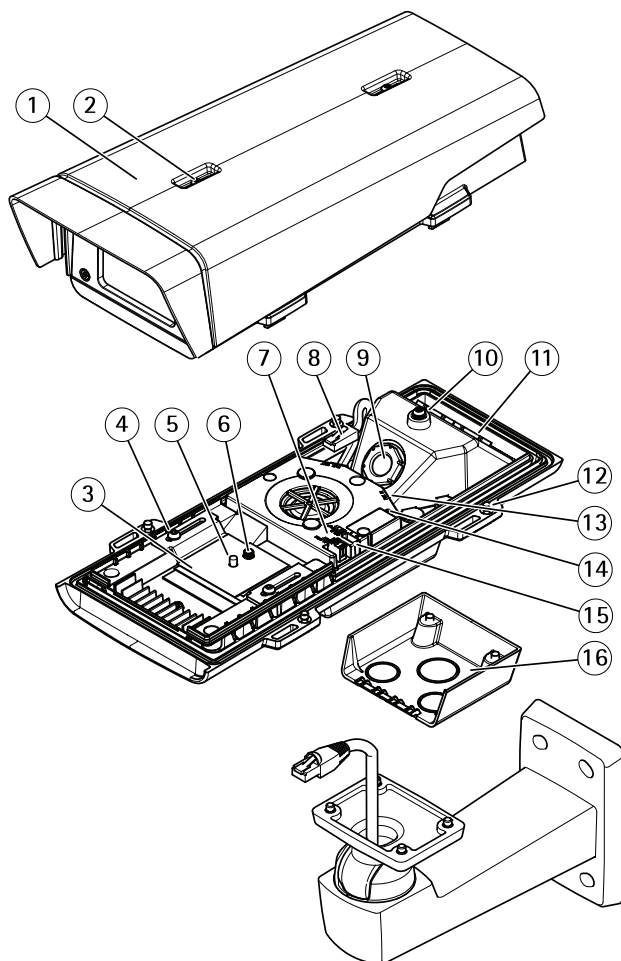
Carcasa de protección AXIS T92E20
