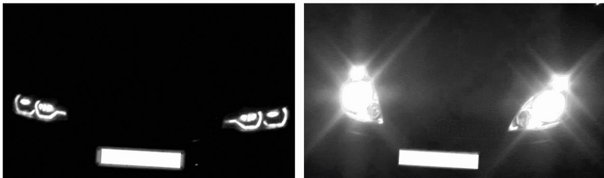
Figure 16. Слева: ИК фильтр задерживает свет светодиодных фар, эффективно снижая засветку и паразитные отражения в объективе. Справа: свет галогенных фар проходит через ИК фильтр, образуя засветку в объективе. Эти два изображения были сняты почти одновременно, с одинаковыми настройками и ориентацией камеры, одной и той же камерой с ИК фильтром.
