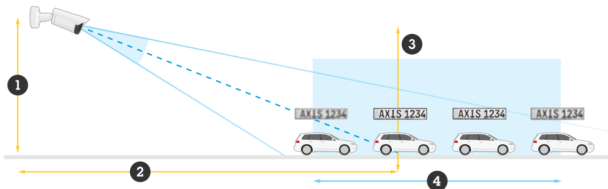
Figure 11. 1: высота, 2: расстояние съемки или фокусное расстояние, 3: фокальная плоскость, 4: глубина резкости. Глубина резкости определяет диапазон вокруг фокальной плоскости, где изображение обладает достаточной резкостью.
