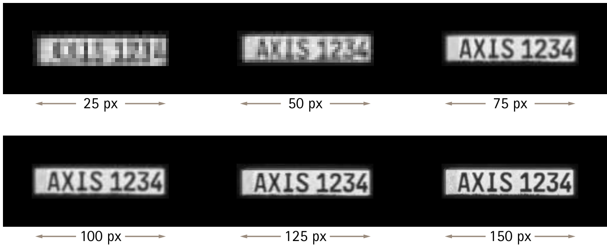
Figure 4. Чтобы буквы на изображении имели полную контрастность, стандартный европейский номерной знак должен занимать не менее 75 пикселей по ширине. Для большинства программных средств распознавания номерных знаков требуется, чтобы номерной знак занимал 100-150 пикселей по ширине.
