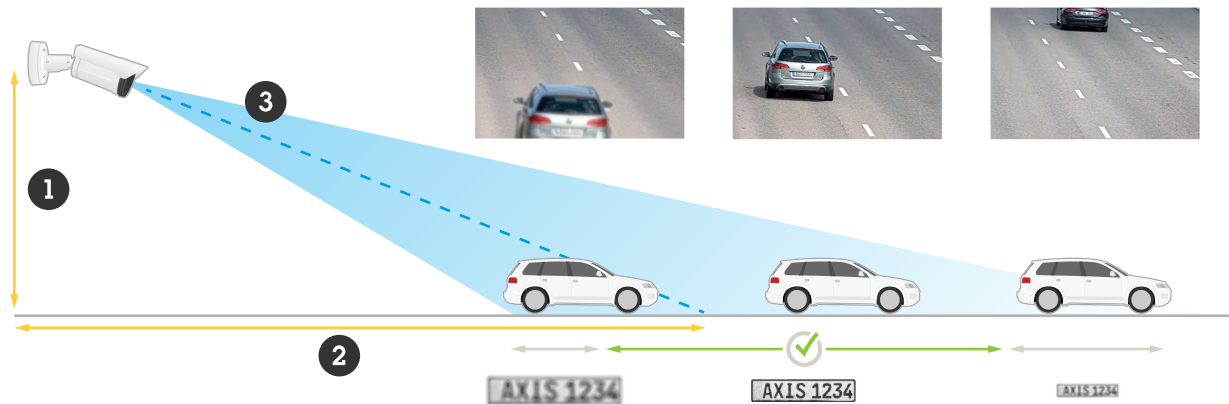
Figure 12. Диапазон обнаружения может быть ограничен глубиной резкости и разрешением. 1: высота, 2: расстояние съемки (фокусное расстояние), 3: угол зрения по вертикали
