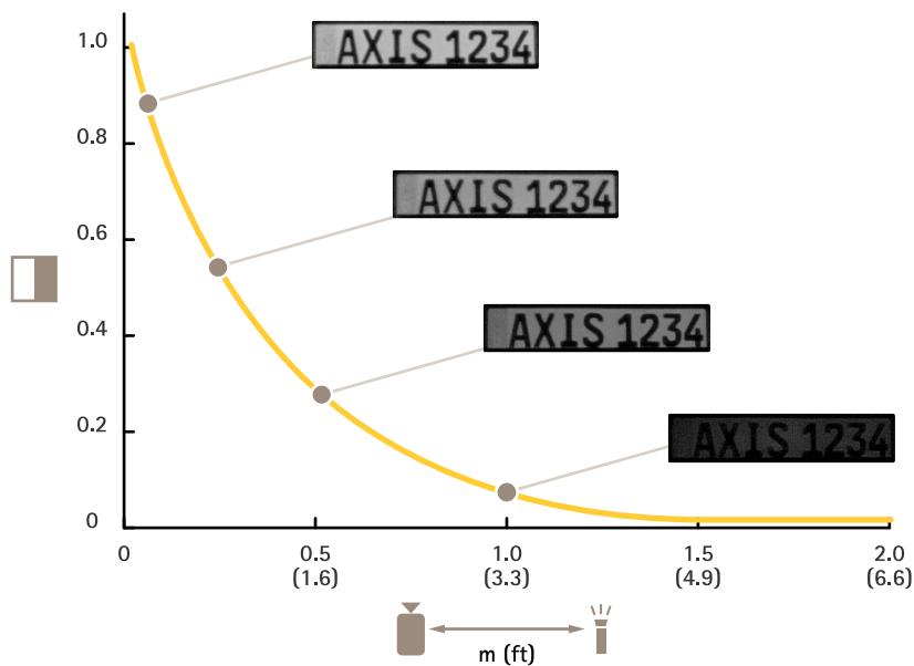
Figure 8. Относительная контрастность номерного знака, находящегося на расстоянии 10 м, как функция расстояния (перпендикулярно оси дороги) между камерой и внешним ИК источником.
