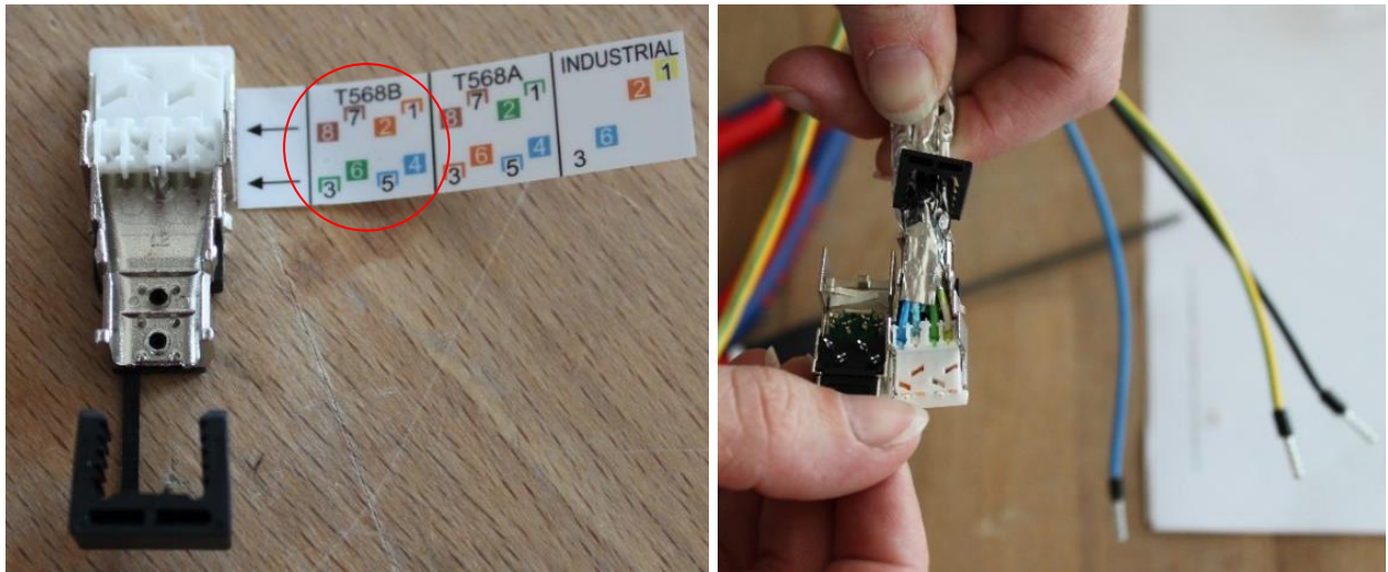
Abb. 4.1 – Auflegen des Steckers
