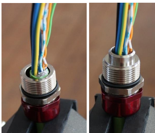
Abb. 3.2 – Konfigurieren der Verbindung für die Kabeldurchführung
