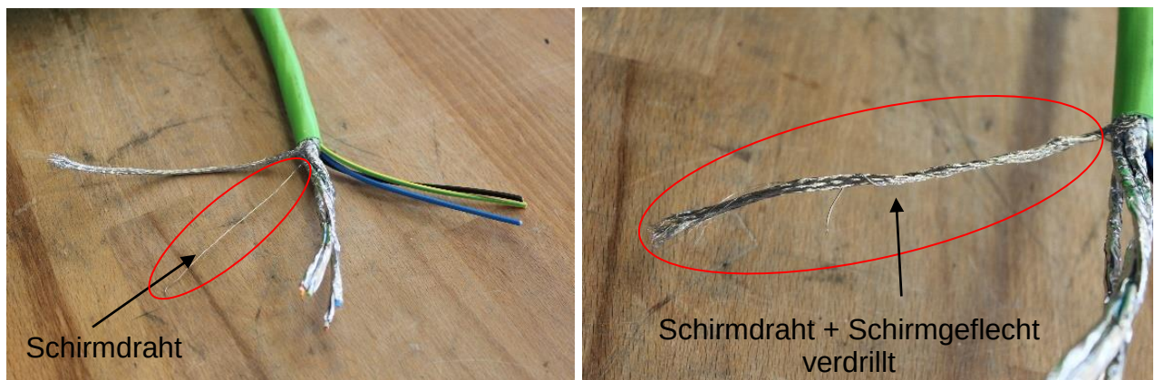
Abb. 2.3 – Schirmdraht und Schirmgeflecht
