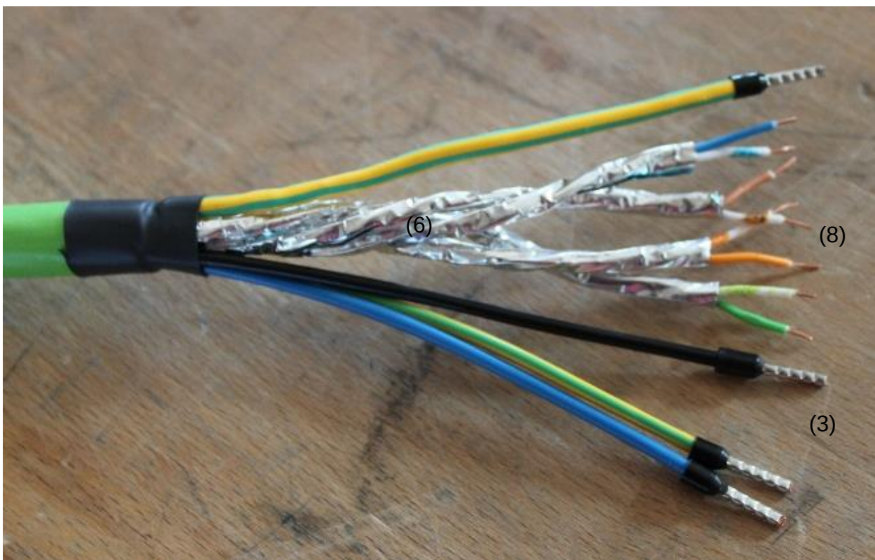
Abb. 2.5 – Fertig konfektioniertes Kabel
