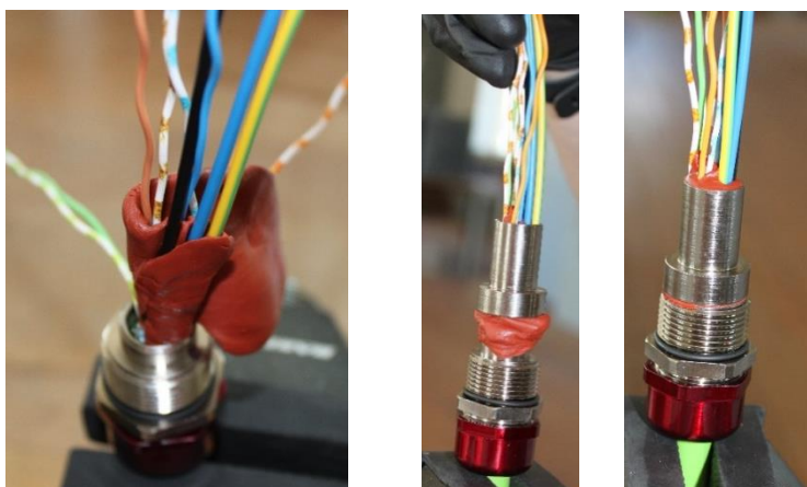
Abb. 3.3 – Verkneten der Kabeldurchführung
