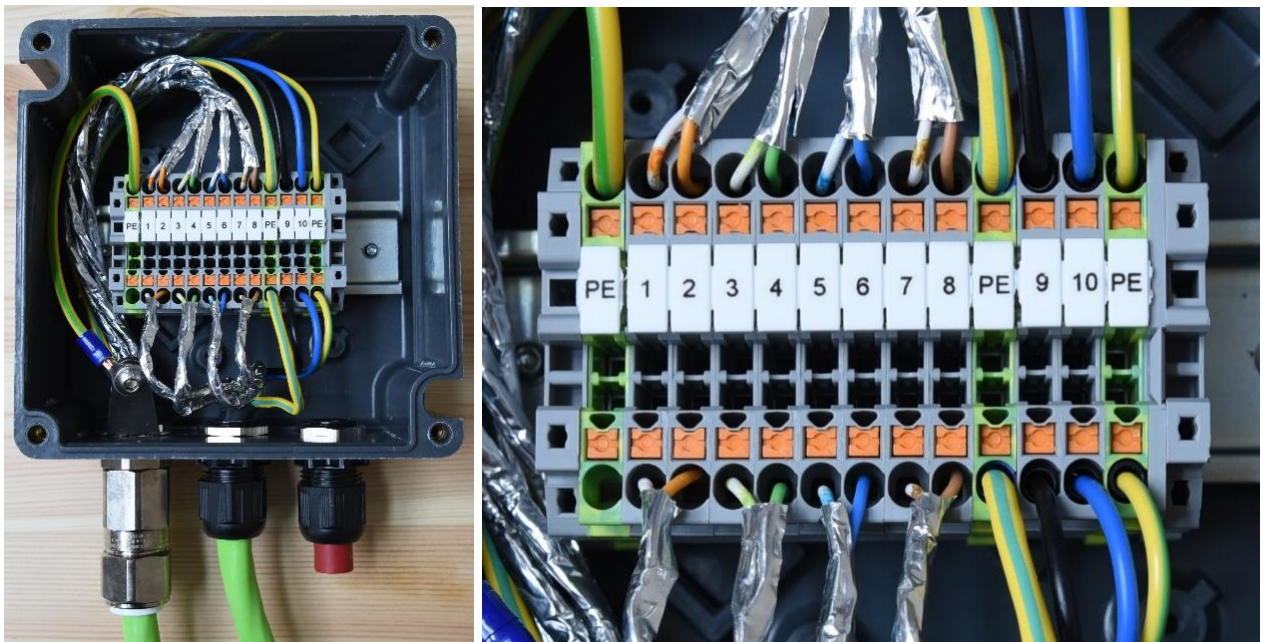
Abb. 2.6 – Verbindung im Klemmkasten
