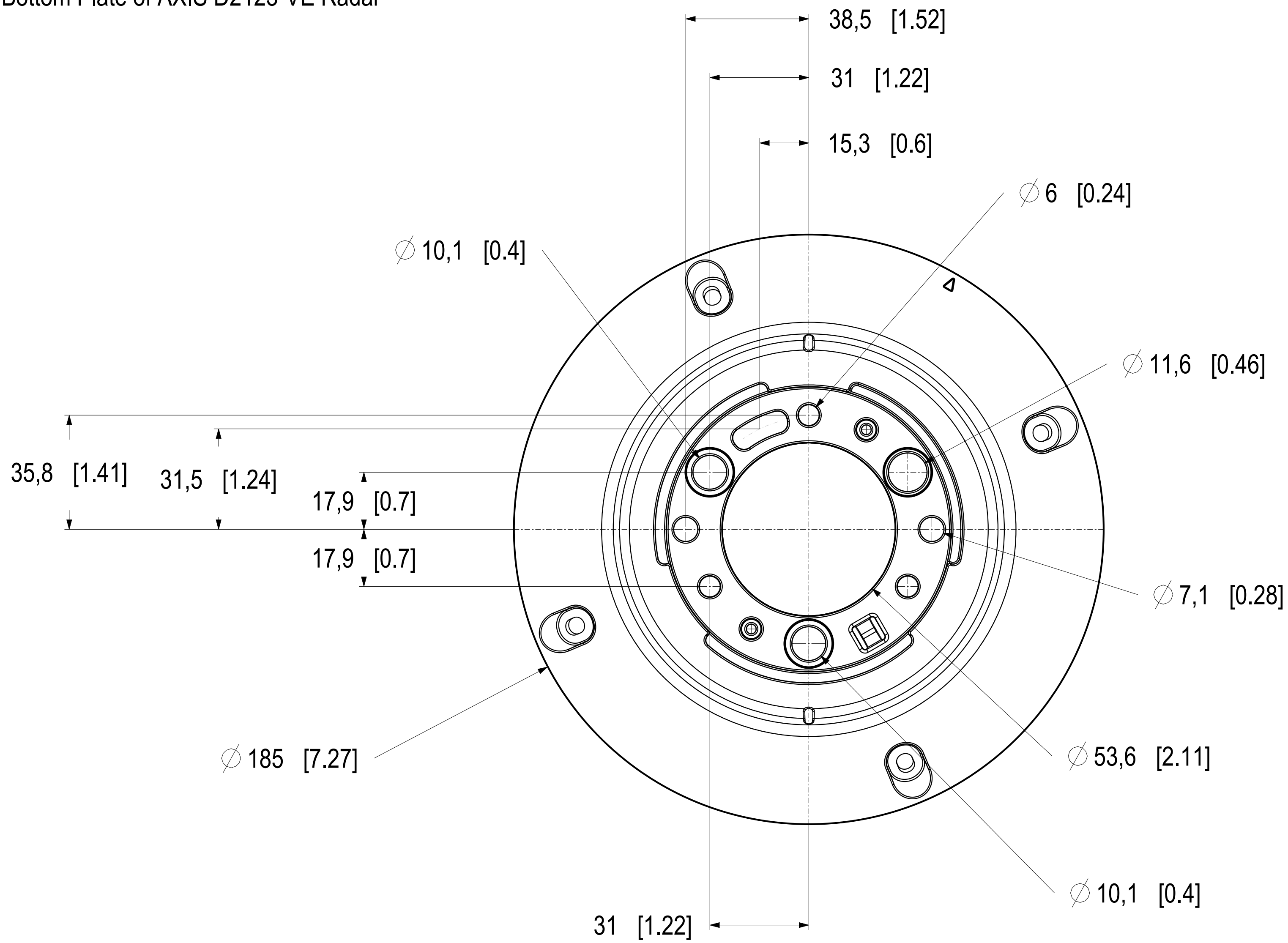
Bottom Plate of AXIS D2123-VE Radar
