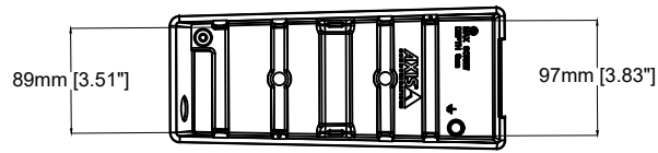
B - B
