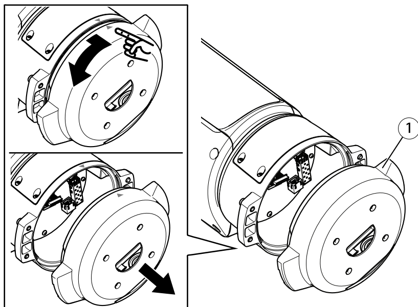
1 底座单元
