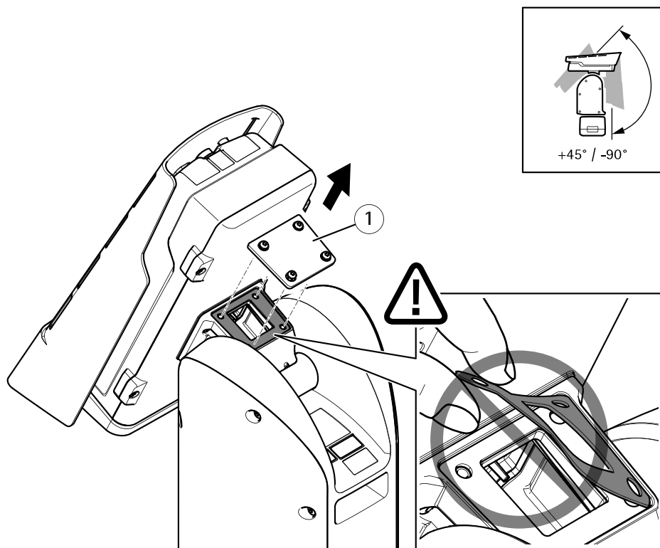
1 Couverture
