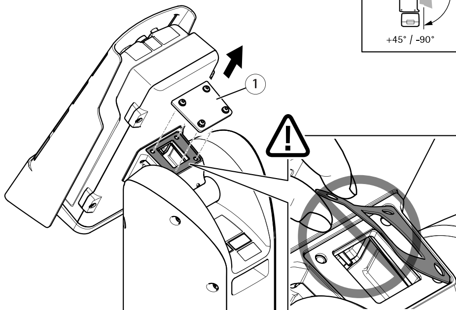
1 Cubierta
