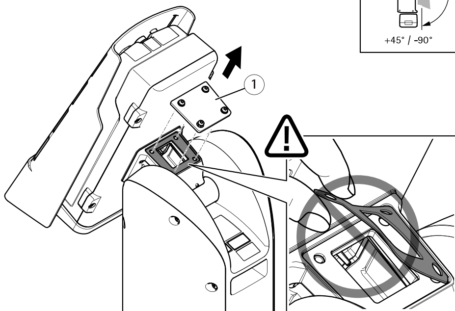
1 カバー
