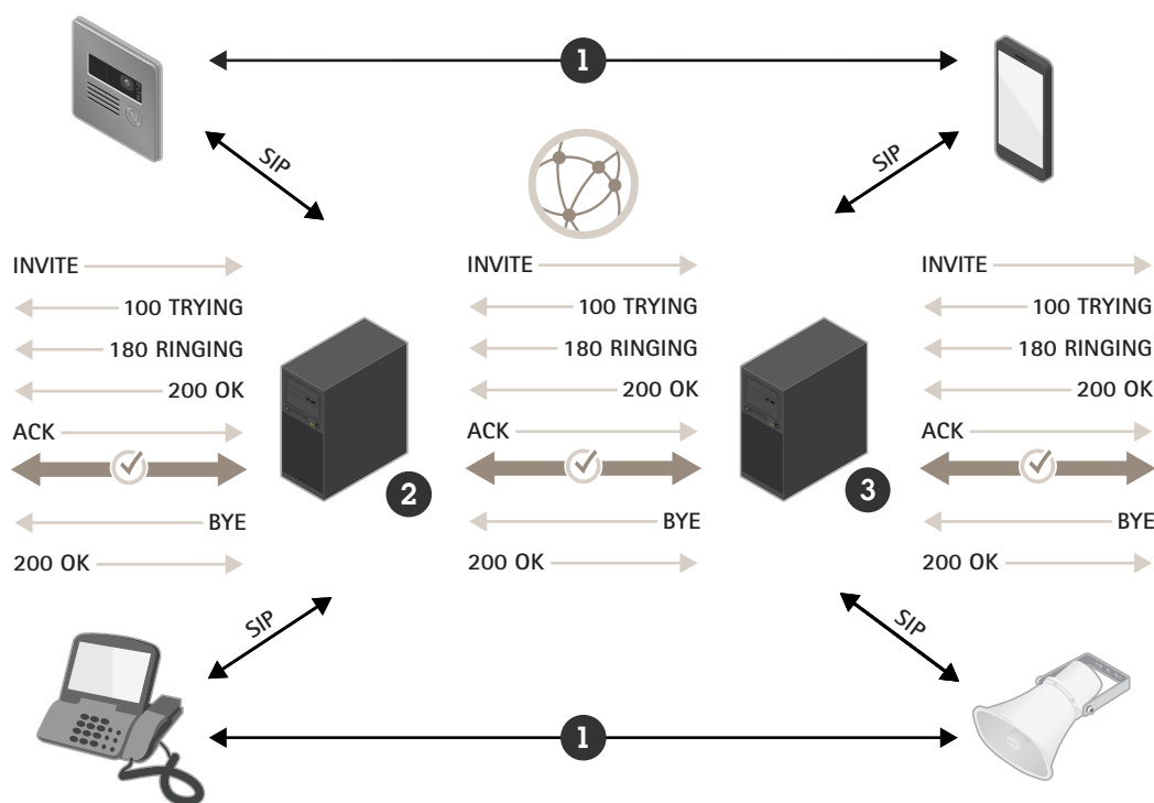
Figure 1. Configurazione di una chiamata in un'infrastruttura SIP complessa. I flussi multimediali RTP (1) viaggiano direttamente tra le parti una volta impostata la sessione SIP tra l'iniziatore (2) e il destinatario (3).
