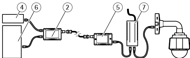
Beispiel 3: Externe Netzteilösung zusammen mit Midspan
