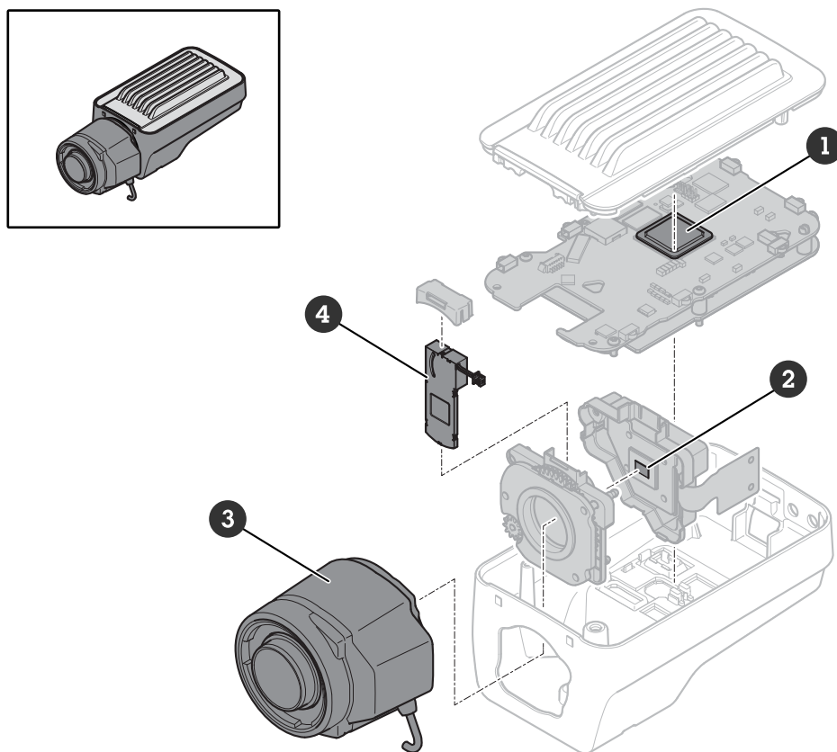
Figure 3. Vista detallada de una cámara de red Axis. En la imagen aparecen resaltados los componentes optimizados por la tecnología Lightfinder: (1) sistema en chip con módulo de procesamiento de señal de imagen (ISP) integrado, (2) sensor de imagen, (3) objetivo y (4) filtros.
