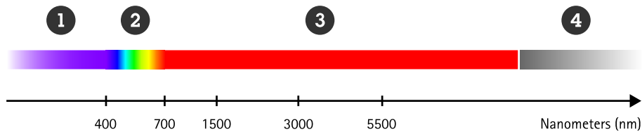
Figure 1. Parte del espectro electromagnético con los intervalos de energía marcados en longitudes de onda (nanómetros). Los intervalos de energía, de izquierda a derecha, son: (1) luz ultravioleta, (2) luz visible, (3) luz infrarroja, (4) microonda.
