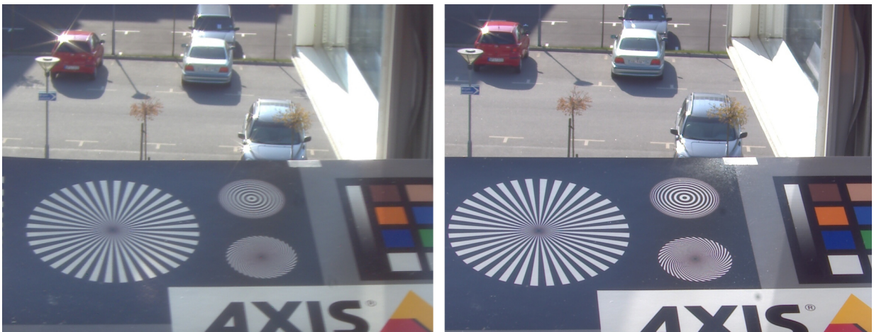
左图采用直流驱动光圈 (DC-Iris) 镜头拍摄。右图采用精确光圈 (P-Iris) 镜头拍摄，对比度比左图更高。
