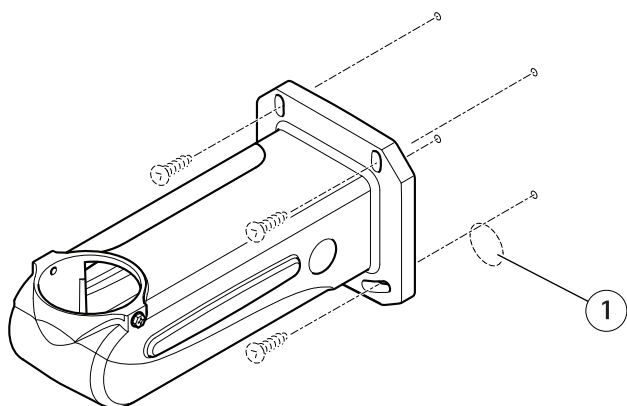
1 ケーブル孔
