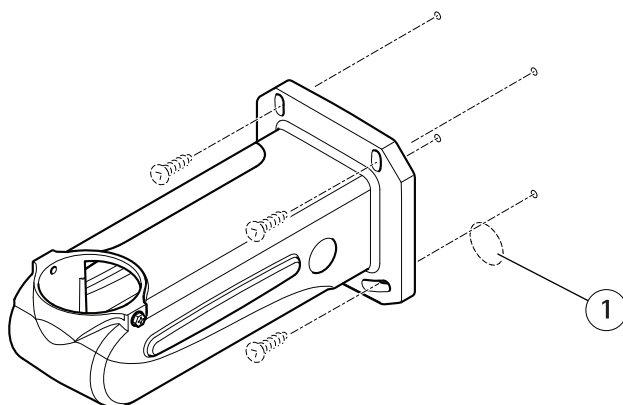
1 电缆孔
