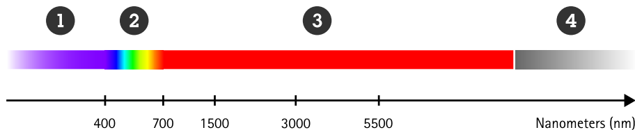
Figure 1. Część widma promieniowania elektromagnetycznego z zakresami energii oznaczonymi długościami fal (w nanometrach). Zakresy energii od lewej do prawej: (1) promieniowanie nadfioletowe, (2) światło widzialne, (3) promieniowanie podczerwone, (4) mikrofałe.
