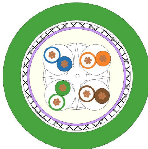
Илл. 2-1 Изображение в разрезе: SKD04-T .flex
