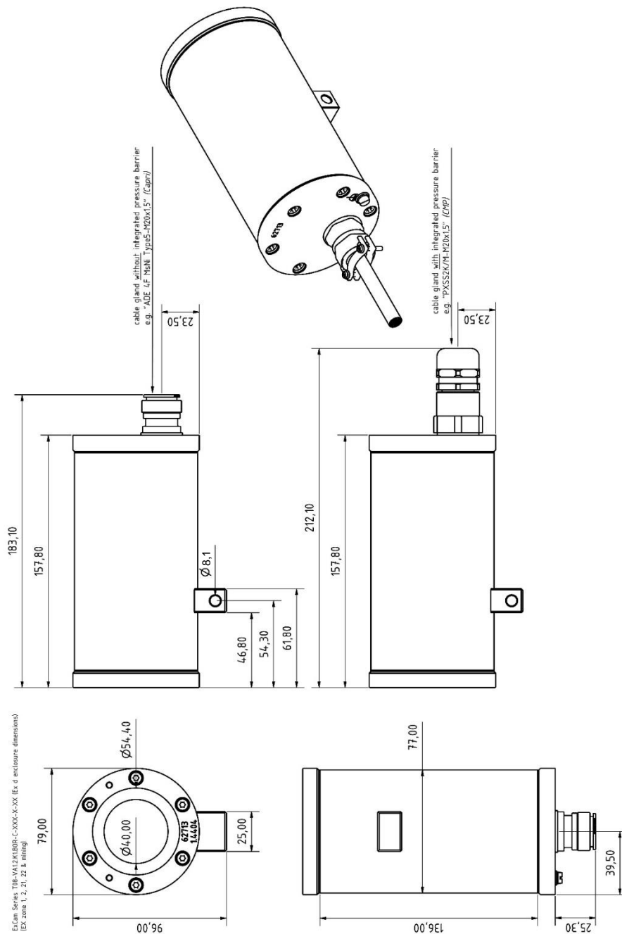
Илл. 10.1 – Размеры T08 ExCam XF M3016
