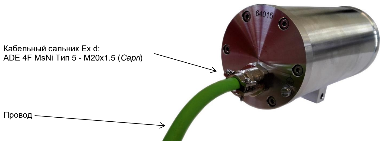
Илл. 5.2 – Кабельный сальник Ex d и подвод энергии
