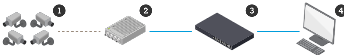
Figure 1. 模拟摄像机 (1) 可以使用传统的同轴电缆连接到视频编码器 (2)。视频编码器对视频进行数字化处理，然后通过局域网将其发送到网络交换机 (3)，交换机再将其传递给视频管理软件 (VMS) (4)。
