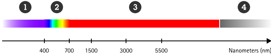
Figure 1. 파장(nm)으로 표시된 에너지 범위의 전자기 스펙트럼 일부. 에너지 범위는 왼쪽에서 오른쪽으로 (1) 자외선, (2) 가시광선, (3) 적외선, (4) 마이크로웨이브입니다.
