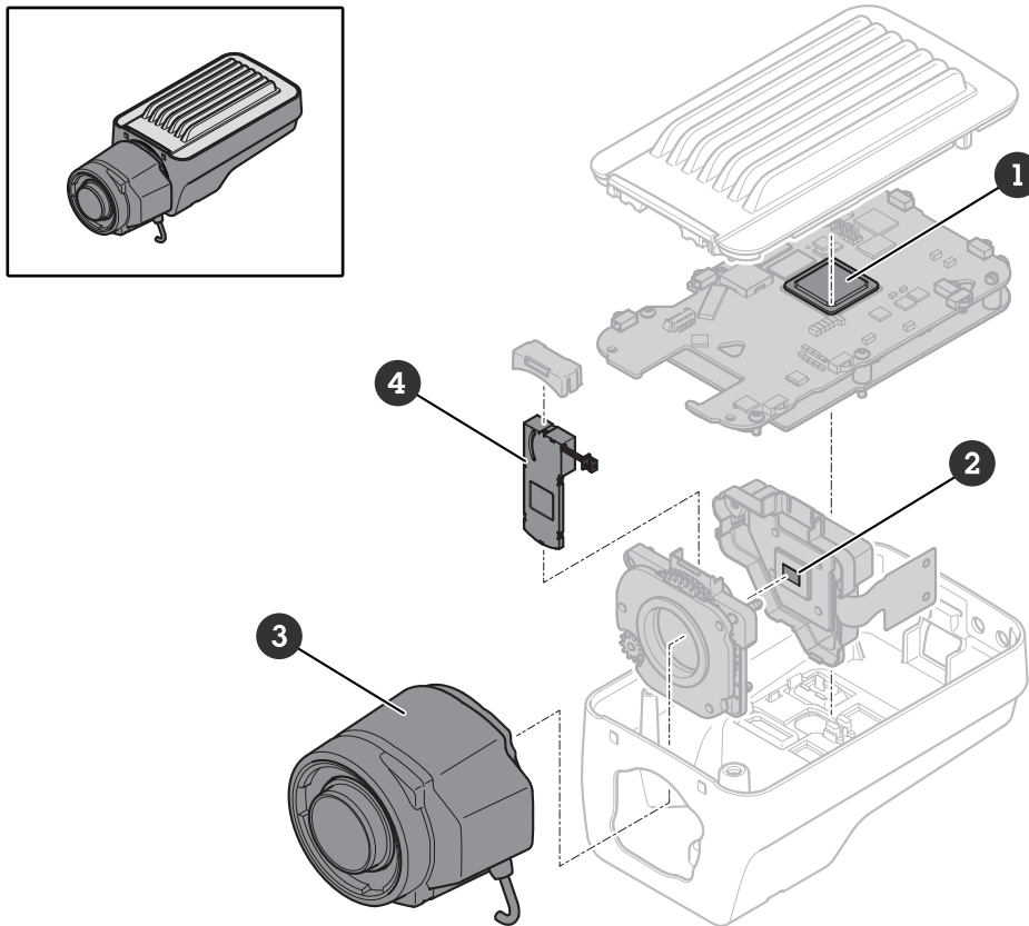
Figure 3. Axis 네트워크 카메라의 분해도. 강조 표시된 부품은 Lightfinder 기술에 최적화된 부품으로, (1) 이미지 신호 처리(ISP) 모듈이 내장된 시스템 온 칩, (2) 이미지 센서, (3) 렌즈, (4) 필터입니다.
