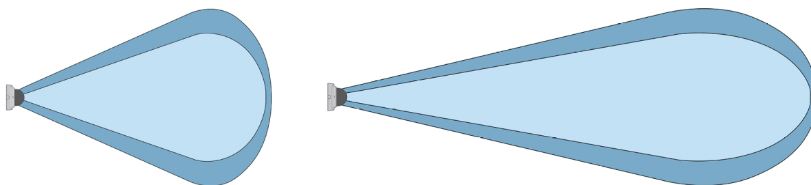
Figure 7. Dans certaines caméras, OptimizedIR contrôle l'angle d'éclairage IR pour suivre les ajustements effectués dans le champ de vision de la caméra.
