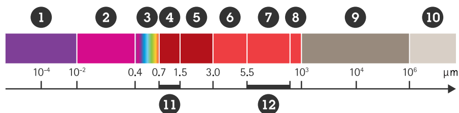
Figure 1. Le spectre du rayonnement électromagnétique. Les éclairages IR fonctionnent dans la région de l'infrarouge proche (11) et les caméras thermiques dans la région des grandes longueurs d'onde IR (12).
