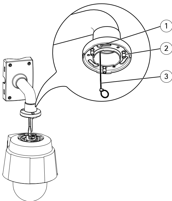
安装示例（墙挂支架单独出售）
