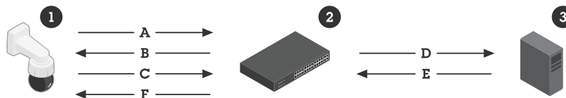
Figure 8. Descripción más detallada del proceso de onboarding. IEEE 802.1AR para la identidad segura del dispositivo define un método para identificar un dispositivo (1) a través de peticiones IEEE 802.1X EAP (EAP-TLS) usando un servidor RADIUS (3) para dar acceso al dispositivo a la red.
