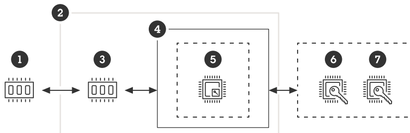
Figure 11. Los dispositivos con Axis Edge Vault tienen módulos de computación criptográfica de hardware (elemento seguro (6) y TPM (7)) que están montados en la placa base justo al lado del procesador principal del SoC (4). El TEE (5) es un área segura del propio procesador principal del SoC. La ROM de arranque integrada
