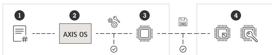
Figure 12. Uso de módulos de hardware y software criptográficos conformes con FIPS 140 en un dispositivo Axis. Para las aplicaciones (1) se utiliza el módulo criptográfico de Axis, integrado en el AXIS OS (2) del dispositivo Axis. El módulo criptográfico de Axis lleva a cabo las operaciones criptográficas, tanto simétricas como asimétricas, utilizando el SoC (3) y/o los módulos (4) de computación criptográfica basados en hardware integrados para el almacenamiento seguro de claves.
