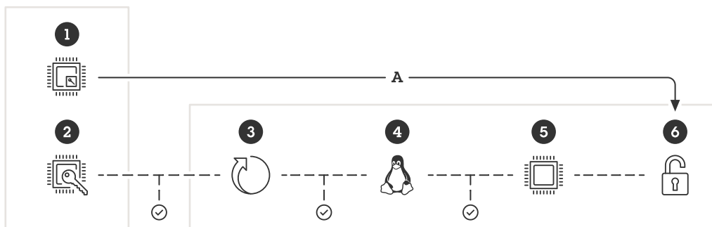
Figure 14. El TEE (1) y el ROM de arranque (2) están integrados en el SoC. Durante el proceso de arranque, se descifra (mediante el TEE) el sistema de archivos de lectura/escritura (6), lo que permite montar el sistema de archivos para que el dispositivo Axis pueda usarlo. En el proceso de arranque se verifica cada parte de la cadena, esto es, el cargador de arranque (3), el kernel de Linux (4) y el sistema de archivos raíz (5), y se autentica el siguiente subsistema en la memoria flash. El resultado final es un sistema de archivos raíz verificado.
