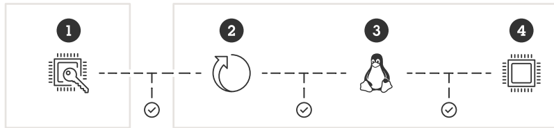
Figure 1. En el proceso de arranque seguro, cada parte de la cadena autentica la siguiente. El resultado final es un sistema de archivos raíz verificado.
