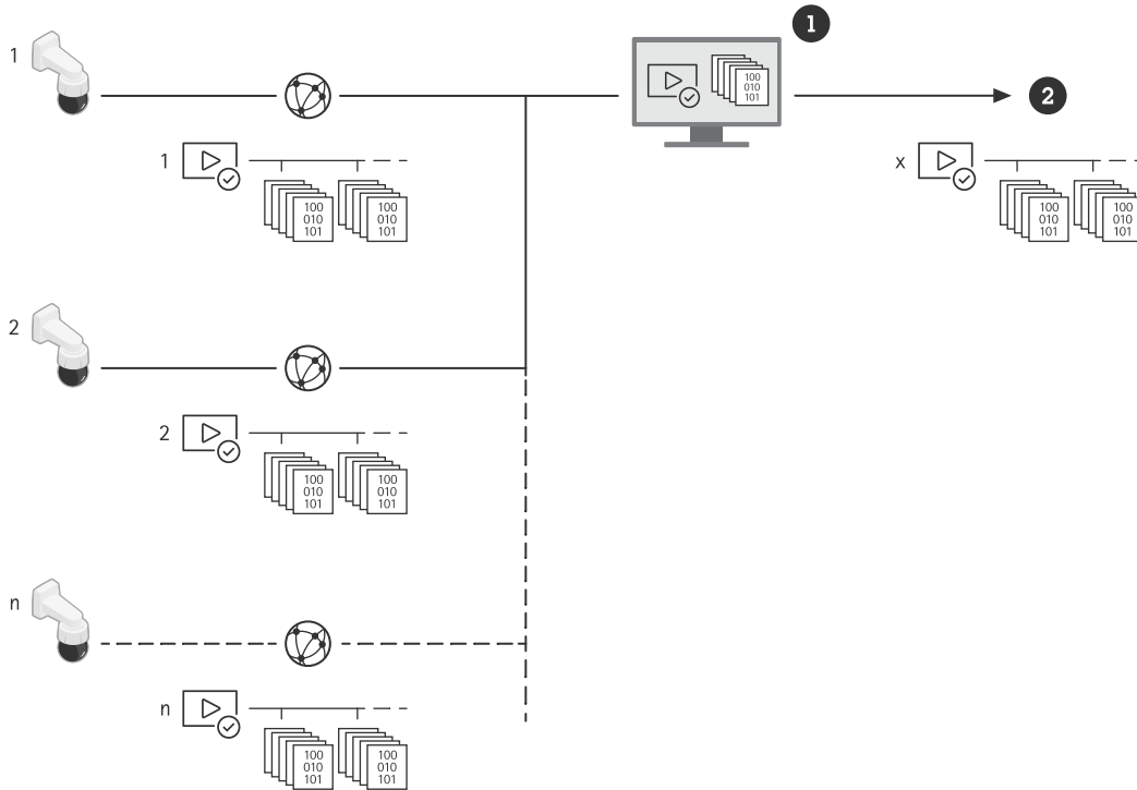
Figure 16. La firma se añade en la propia cámara, lo que permite verificar el contenido en todas y cada una de las fases, desde la fuente hasta el uso final del vídeo.
