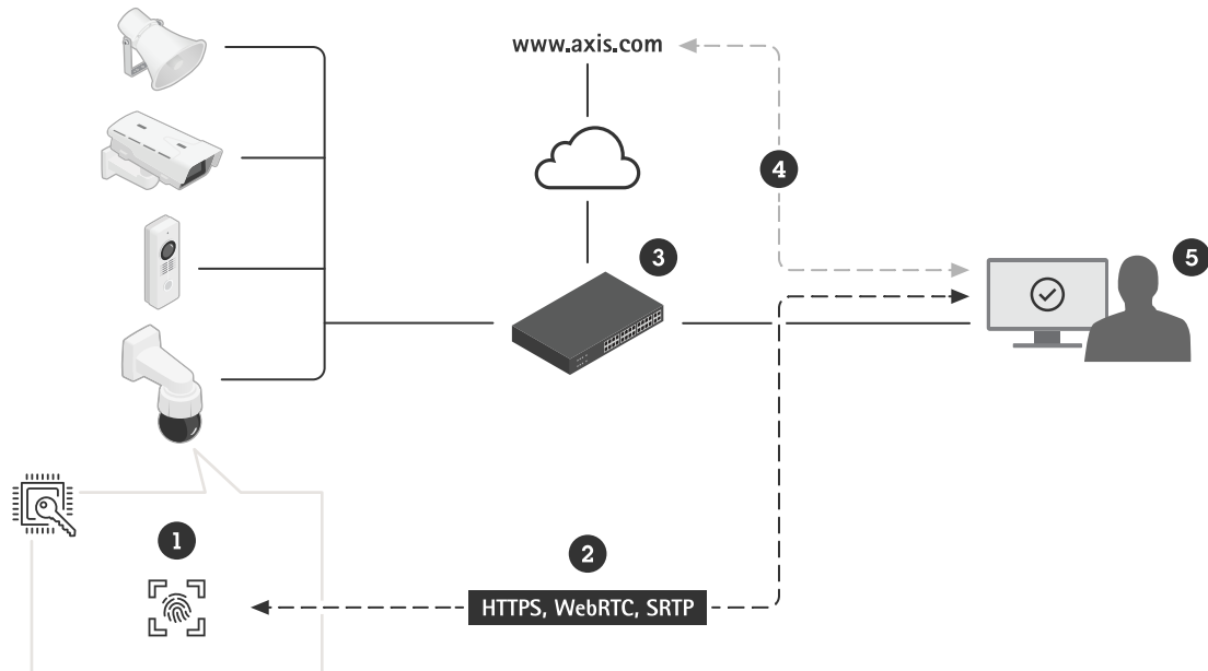
Figure 9. Una vez realizado el onboarding seguro de un dispositivo, las aplicaciones de software (5) de otras partes del sistema pueden usar el ID de dispositivo de Axis (1) y las operaciones criptográficas para verificar y autenticar el dispositivo en distintas comunicaciones a través de TLS (2). El ID de dispositivo de Axis se puede verificar con el certificado de CA raíz del ID de dispositivo de Axis de carácter público (4).
