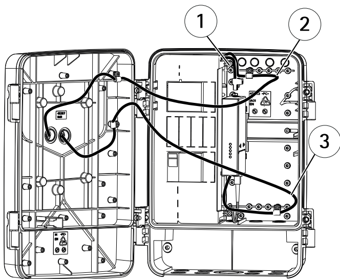
Armoires de convertisseur de média AXIS T98A-VE
