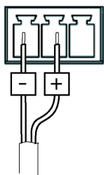
Ingresso alimentazione CC 24-34 V CC AXIS P5522: max 15,5 W
