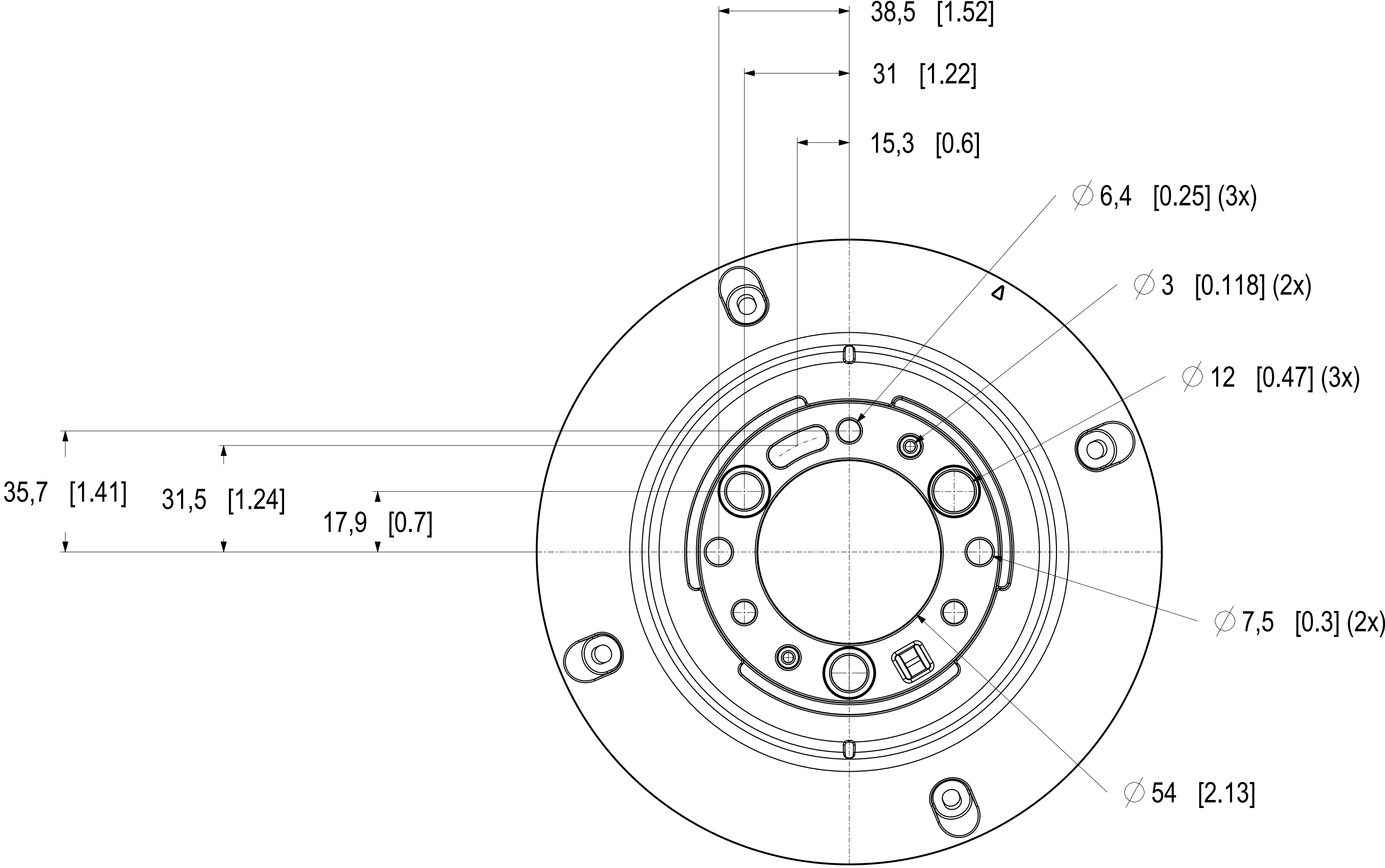
Bottom Plate of AXIS D2123-VE Radar
