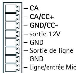
AXIS 233D Connecteur
