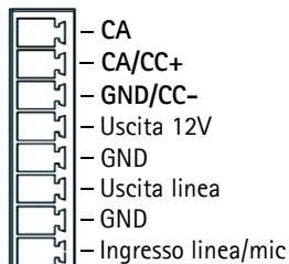
AXIS 233D Connettore
