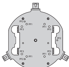
Piastra fissa (vista dal basso)
