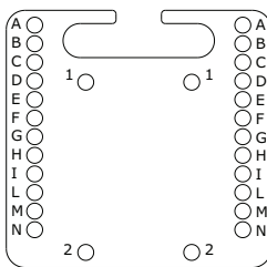
Placa espaciadora
