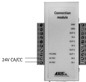
AXIS 233D Connettore
