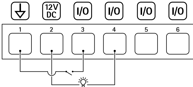
1 Erdung Gleichstrom
