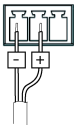
Ingresso alimentazione CC, 24-34 V CC AXIS P5512: max 15,7 W
