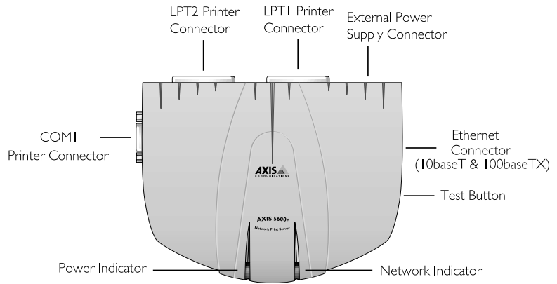
Vue en plan du serveur AXIS 5600+
