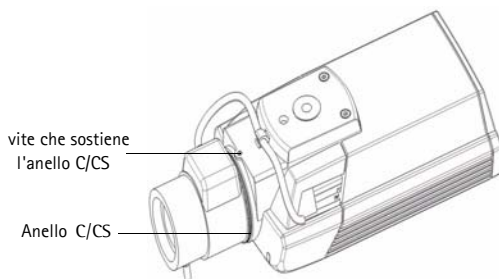
Parte sottostante della telecamera
